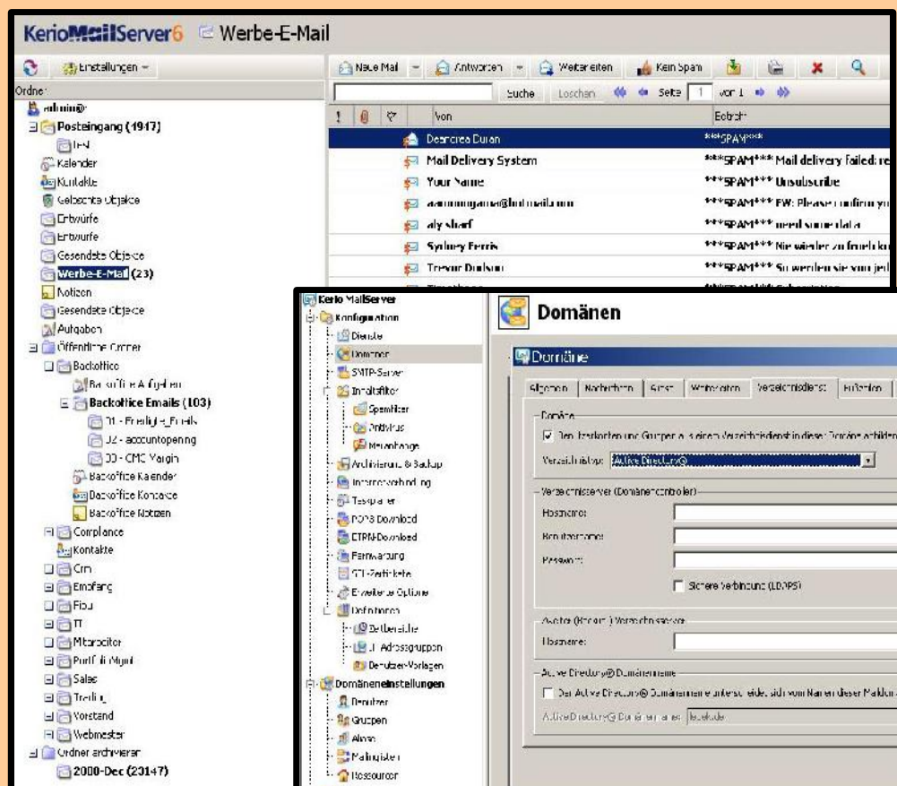
Kerio Web-Interface
